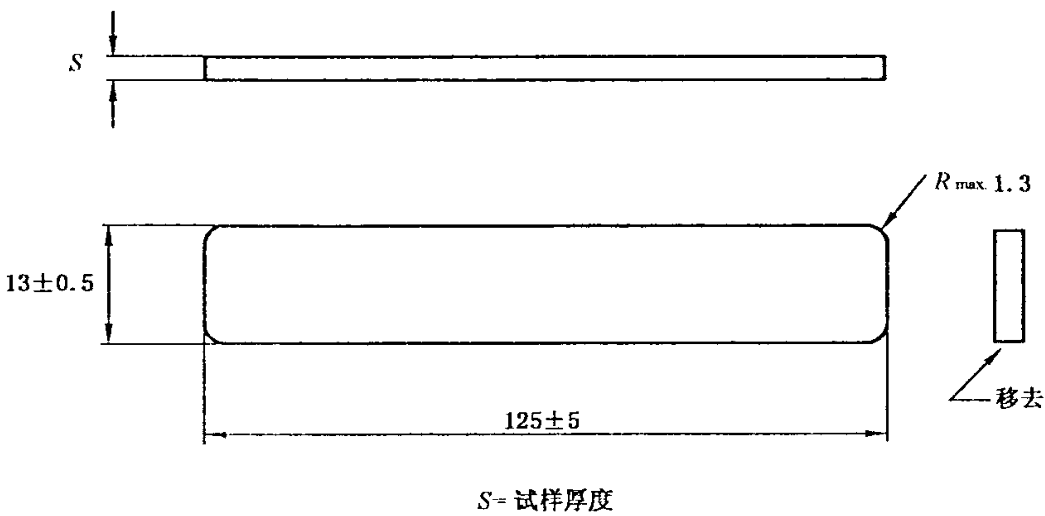
图 4 条状试样
